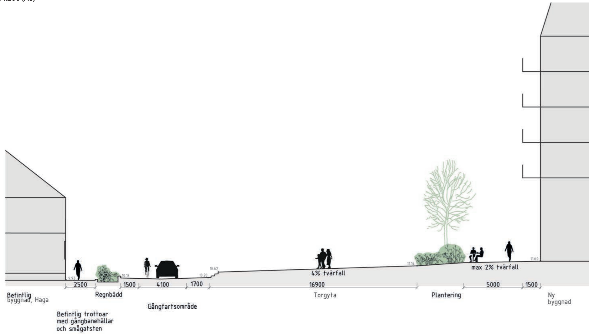
Elevation C-c Skala 1:200/A3
